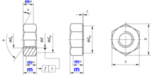
Écrou
