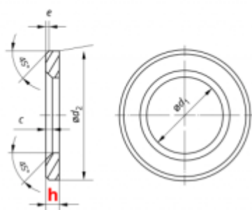
Rondelles
